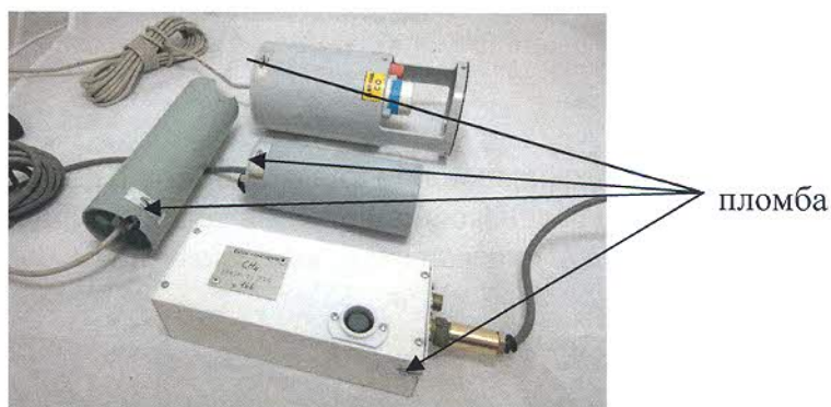
Рисунок 1 – Общий вид блоков датчиков переносных газоанализаторов, схема пломбировки от несанкционированного доступа
