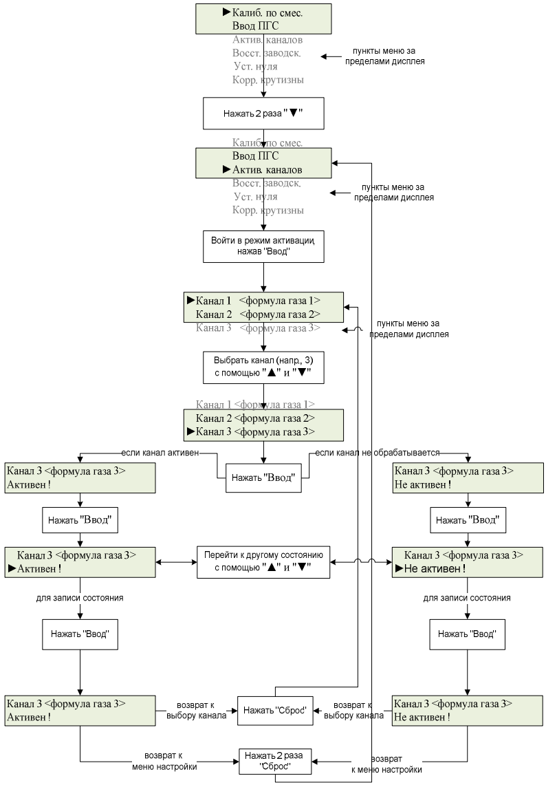
Рисунок 2.1 Активация/деактивация канала
