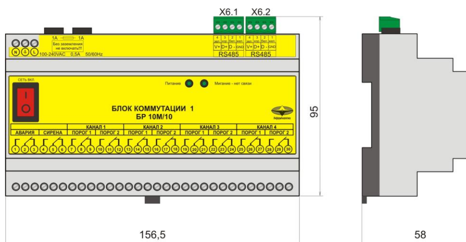
Рис. Е2. Блок коммутации исполнение И22.
